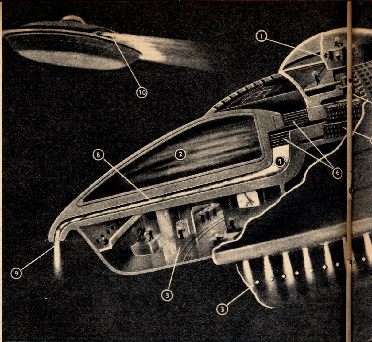
L'Aviazione Militare degli Stati Uniti avrebbe in progetto la costruzione di un nuovo tipo di macchina volante a forma di disco. Il disegno illustra sommariamente le probabili caratteristiche dell'aereo del futuro: 1) cabina di pilotaggio; 2) serbatoio carburante; 3) cabine per l'equipaggio e i passeggeri; 4) albero della turbina centrale; 5) rotor; 6) stabilizzatore di pressione; 7) camera di combustione; 8) tubo di scappamento; 9) fori di uscita dei gas disposti a corona lungo tutta la
