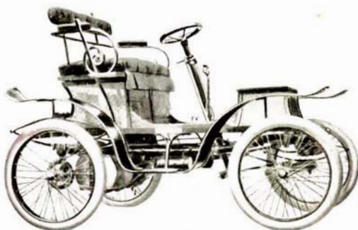
Primo tipo di vettura Bianchi con motore del modello per triciclo ad un cilindro - raffreddamento a mezzo di alette - trasmissione con ingranaggi.
