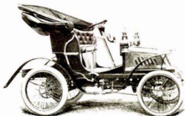
Tipo di vettura Bianchi con motore ad un cilindro della forza di 6 HP - raffreddamento ad acqua per mezzo di una pompa - trasmissione a cardano.
