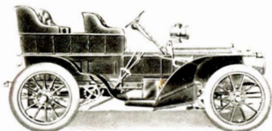
Tipo di vettura Bianchi con motore a quattro cilindri - radiatore a nido d'api - trasmissione a catene - quattro velocità - accensione con magnete a bassa tensione - telaio in lamiera imbottito.
