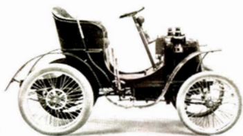
Tipo di vettura Bianchi con motore ad un cilindro della forza di 5 HP - raffreddamento ad acqua per termosifone - trasmissione a cardano.
