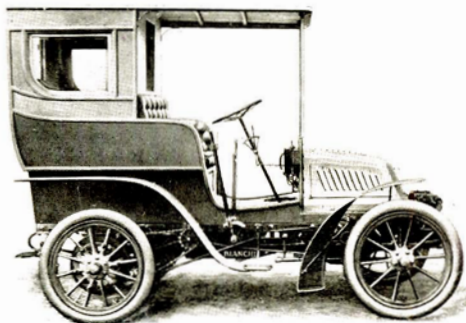
Tipo di vettura Bianchi con motore a due cilindri della forza di 10 HP - trasmissione a catene - raffreddamento per mezzo di una pompa e radiatore ad alette - quattro velocità - telaio in legno armato.
